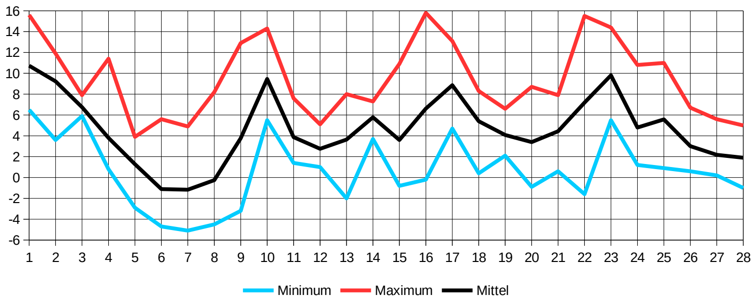
Temperaturen im Februar 2020 (°C)
