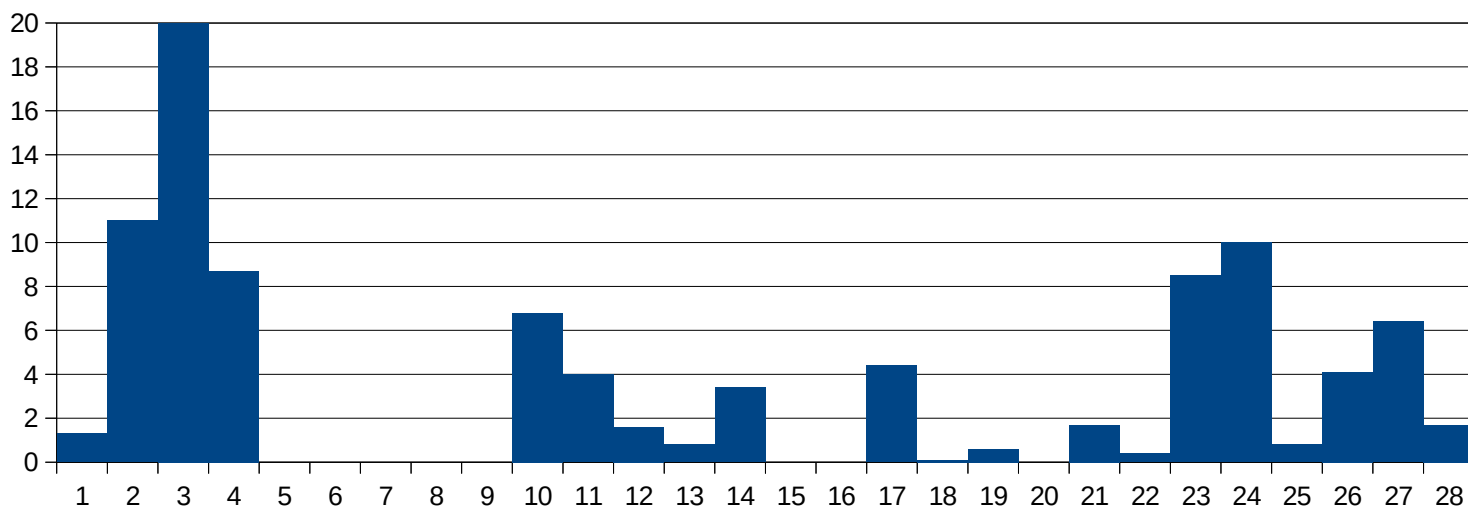
Niederschlag im Februar 2020 (mm)
