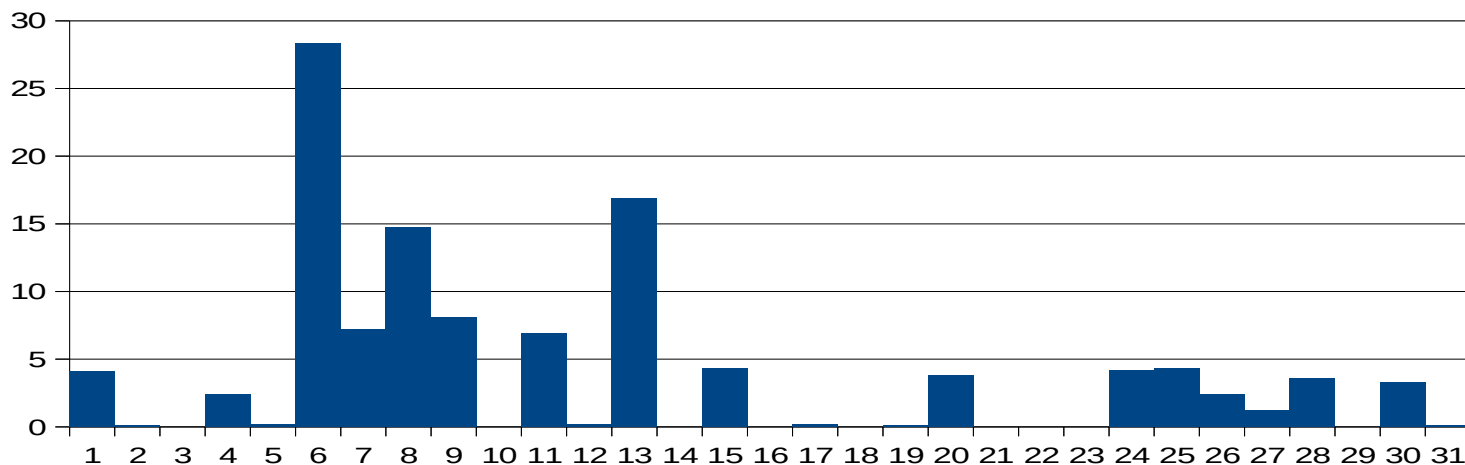
Niederschlag im Juli 2021 (mm)
