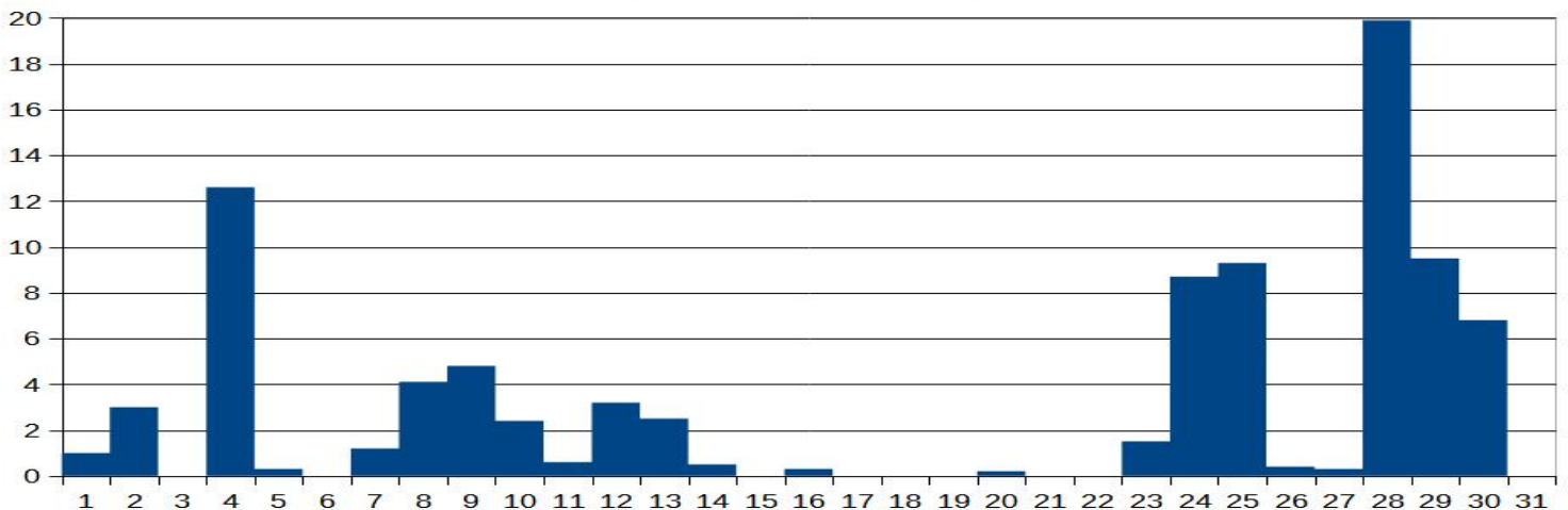
Niederschlag im Dezember 2021 (mm)
